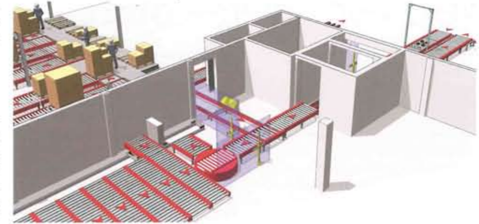
Die Hochregal-Ausgabestationen sind flexibel konzipiert, so dass sie beliebig erweitert und mit Kommissionierplätzen versehen werden können.
